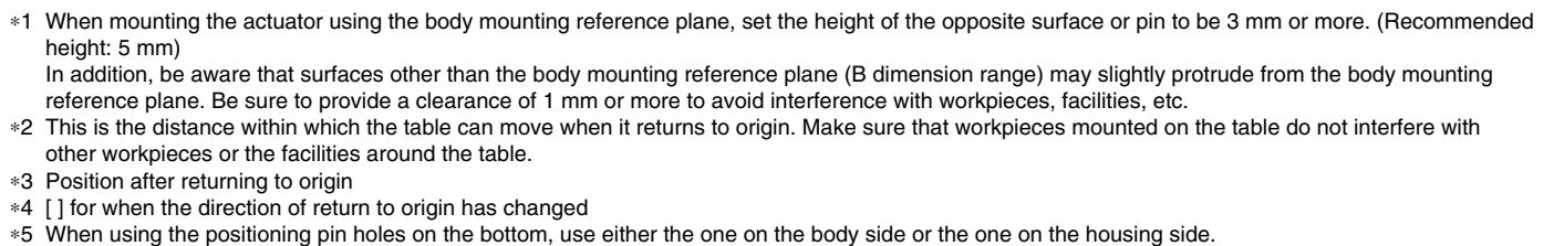
Dimensions
