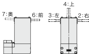
モータ配置:T ケーブル取出し図
