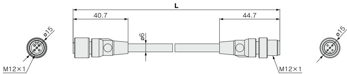
通信ケーブル長さ L
