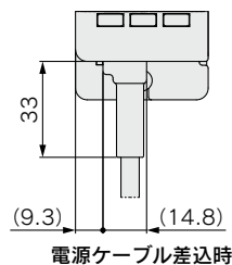
電源ケーブル差込時
