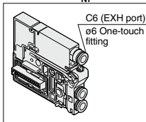
Individual EXH spacer VVQ1000-R-1-C 6 -N 7
