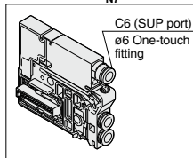
Individual SUP spacer VVQ1000-P-1-C 6 -N 7
