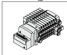
Dual flow fitting assembly VVQ1000-52A-N 9
