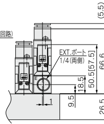
単独EXHスぺーサ取付時の寸法
