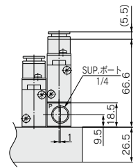
単独SUPスぺーサ取付時の寸法 (SUPポートは、シングルソレノイドの エンドプレート側になります。)
