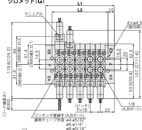
単独EXHスぺーサ取付時の寸法
