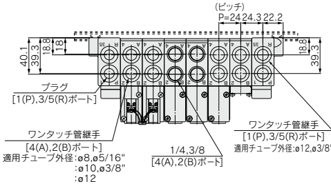
外部パイロット仕様の場合
