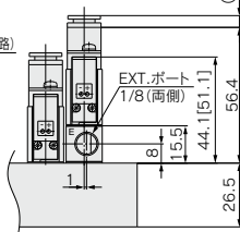
単独EXHスぺーサ取付時の寸法
