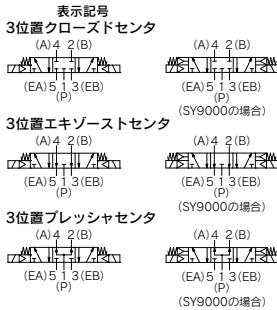
3位置クローズドセンタ/エキゾーストセンタ/プレッシャセンタ
