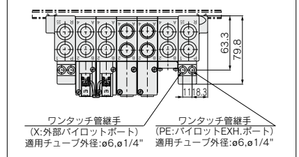
外部パイロット仕様の場合
