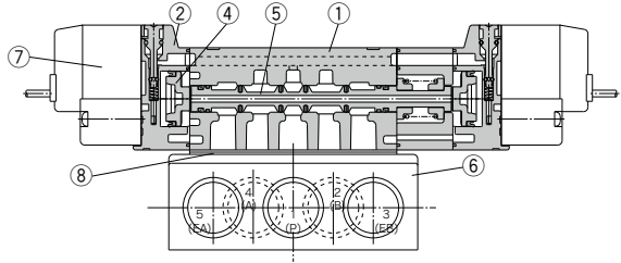
3位置クローズドセンタ/エキゾーストセンタ/プレッシャセンタ
