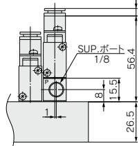
単独SUPスペース取付時の寸法 (SUPポートは、シングルソレノイドの エンドプレート側になります。)
