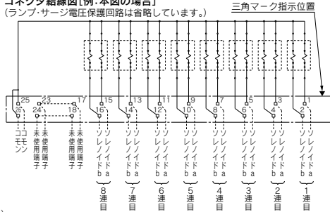
コネクタ結線図[例:本図の場合]
