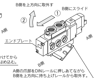
図2.バルブ取外し要領
