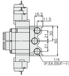
単独EXHスぺーサ取付時の寸法
