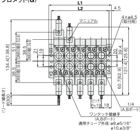
単独EXHスぺーサ取付時の寸法
