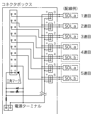
+COM電気回路図
